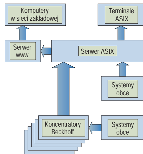
Schemat systemu
